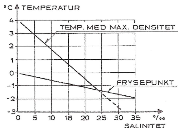
Fig. 5 Frysepunkt og temperatur med maksimal densitet (massefylde) som funktion af temperatur og salinitet (saltindhold) 6
