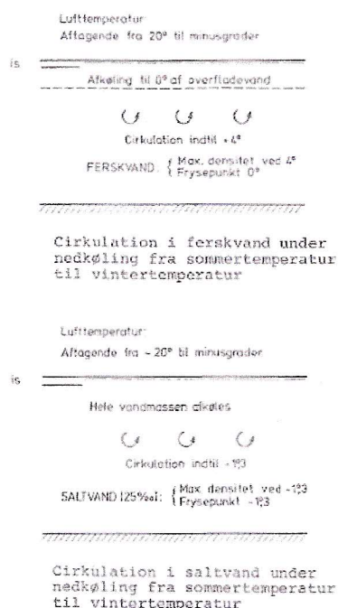
Fig. 6 Vandcirkulation under nedkøling 7
