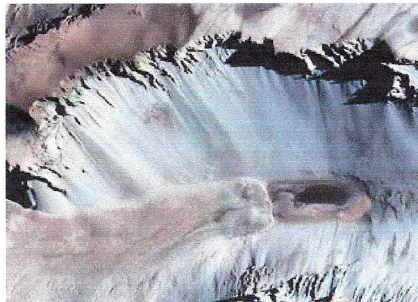
Fig. 4 Don Juan Pond på Antarktis 4
