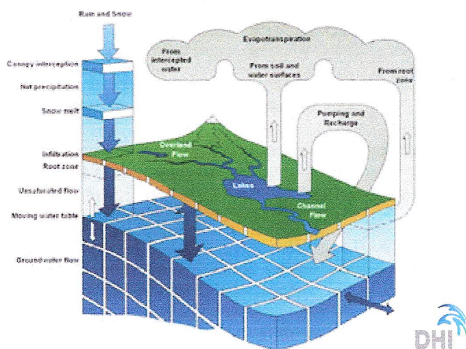
Fig. 2 DHI-model - beskriver vandets bevægelse rundt på Jorden 2
